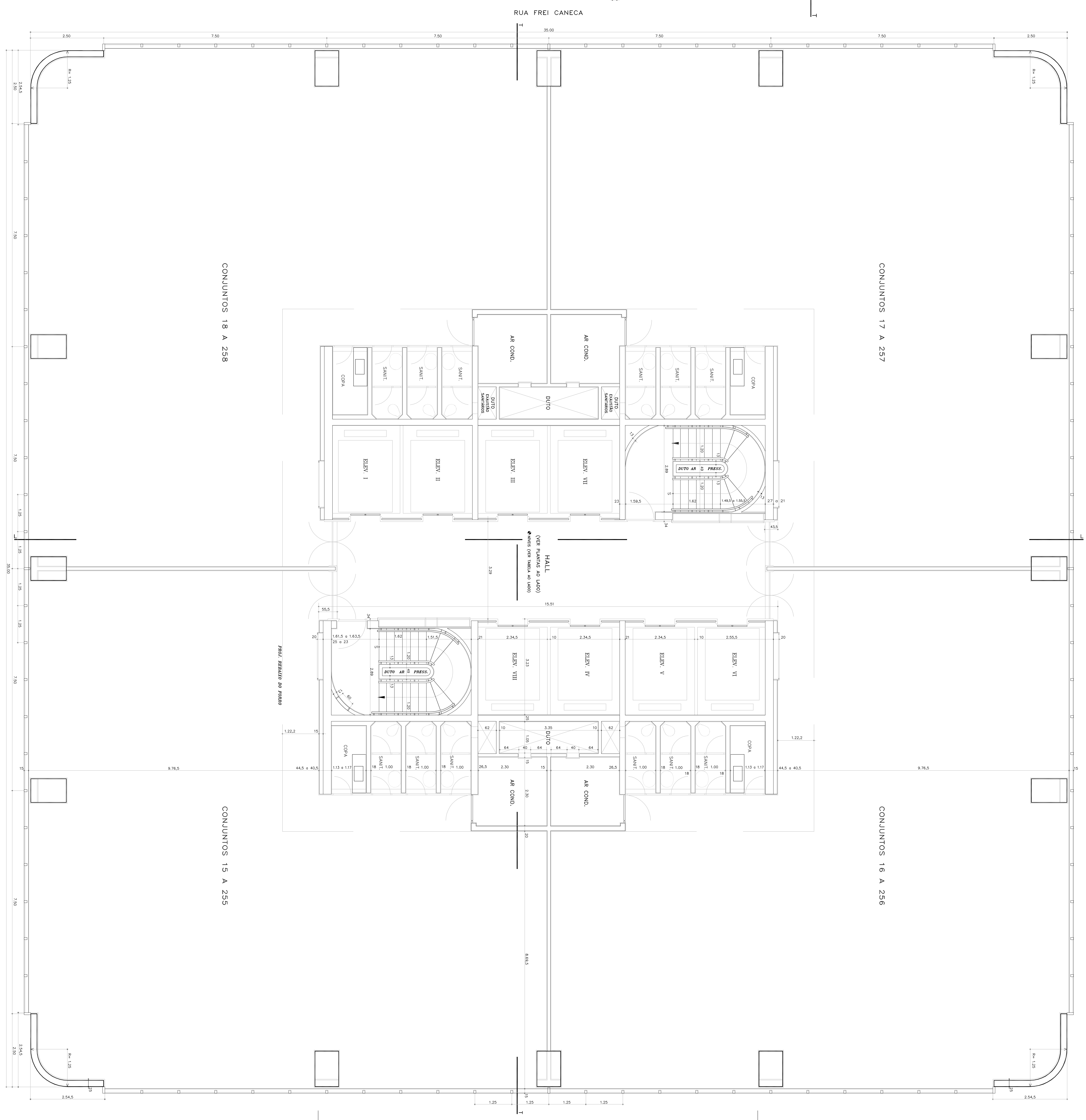
PLANTA DO ANDAR TIPO (1º ao 25º)
